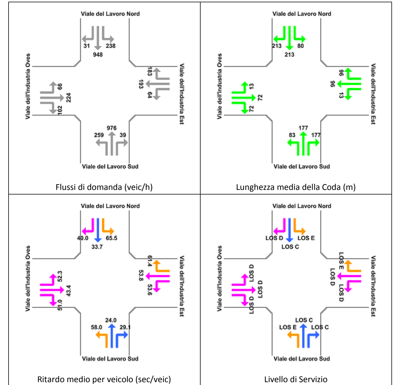
Figura 8-4: Nodo Viale del Lavoro-Viale dell'Industria Risultati delle verifiche - Stato di Fatto Ora di Punta Venerdì 17.00-18.00
