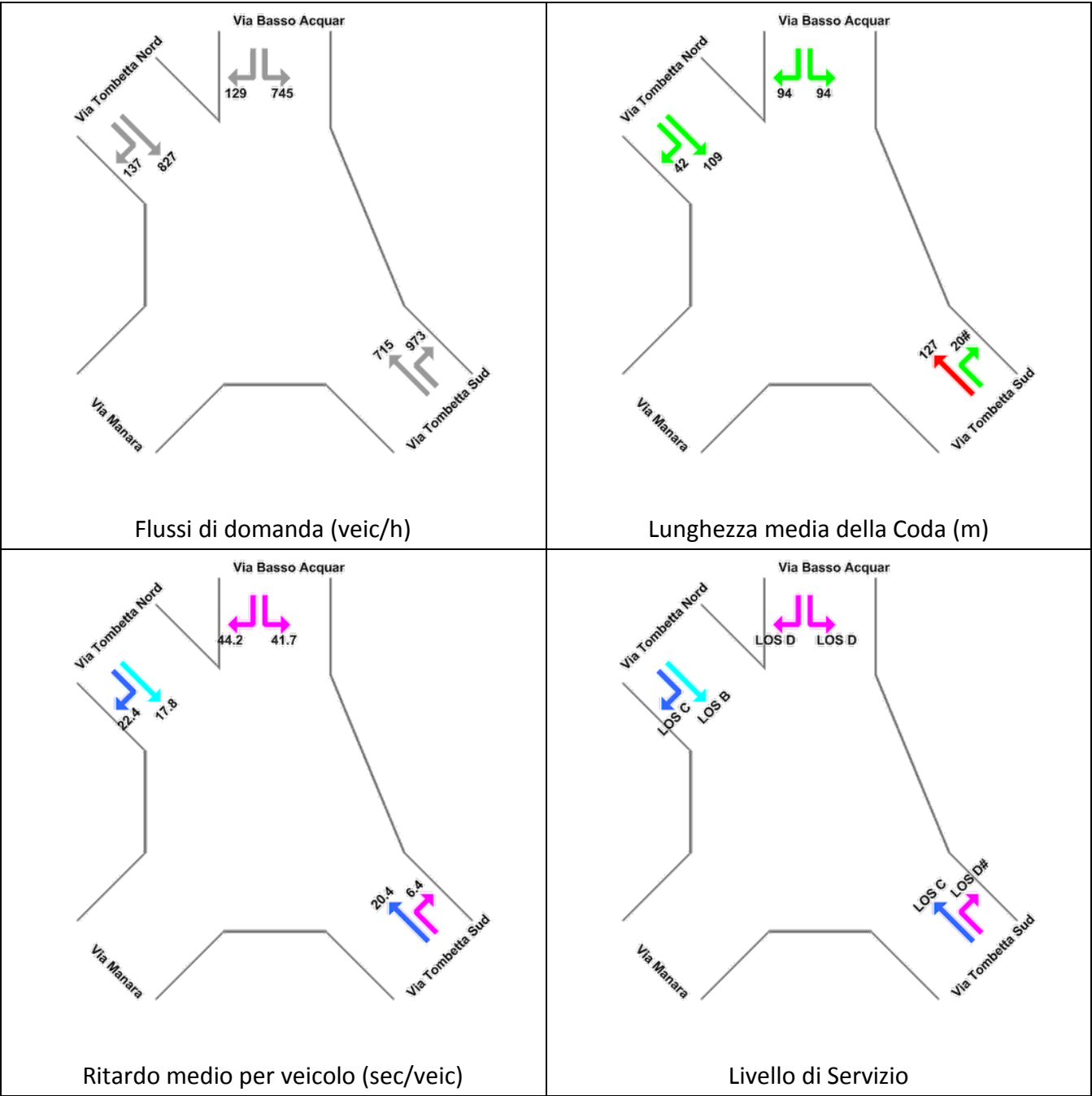
Figura 8-31: Nodo Via Tombetta-Via Basso Acquar Risultati delle verifiche - Stato di Progetto Ora di Punta Venerdì 17.00-18.00
