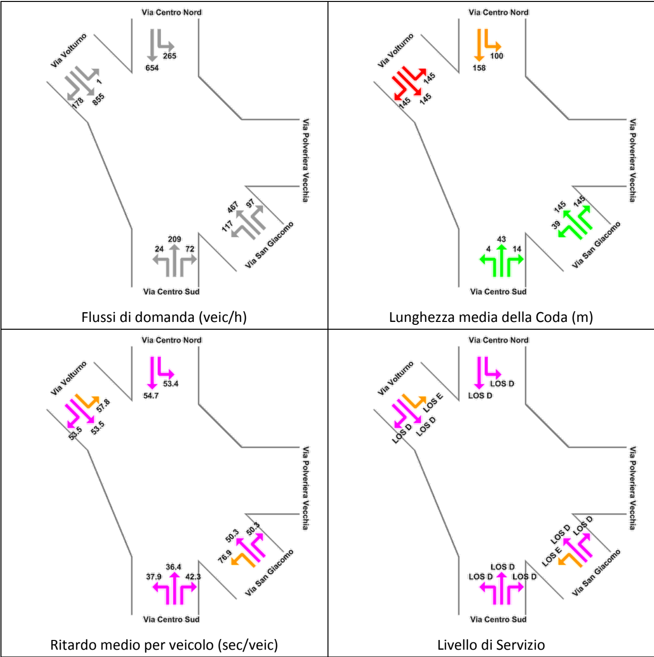
Figura 8-34: Nodo Via San Giacomo-Via Volturmo-Via Centro Risultati delle verifiche - Stato di Fatto Ora di Punta Venerdì 17.00-18.00
