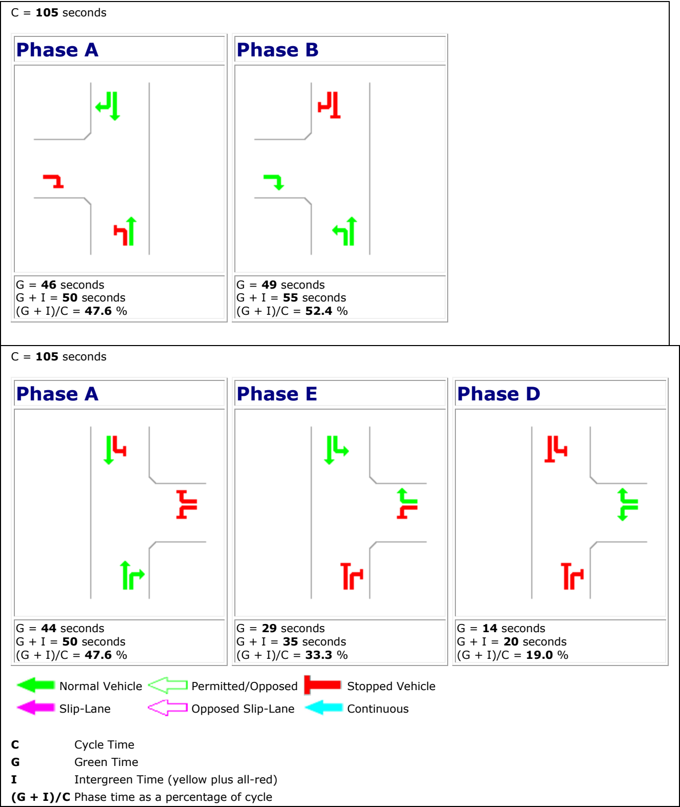
Figura 8-13: Nodo Viale del Lavoro-Viale dell'Agricoltura-Via Scopoli Fasatura impianto semaforico - Stato di Fatto
