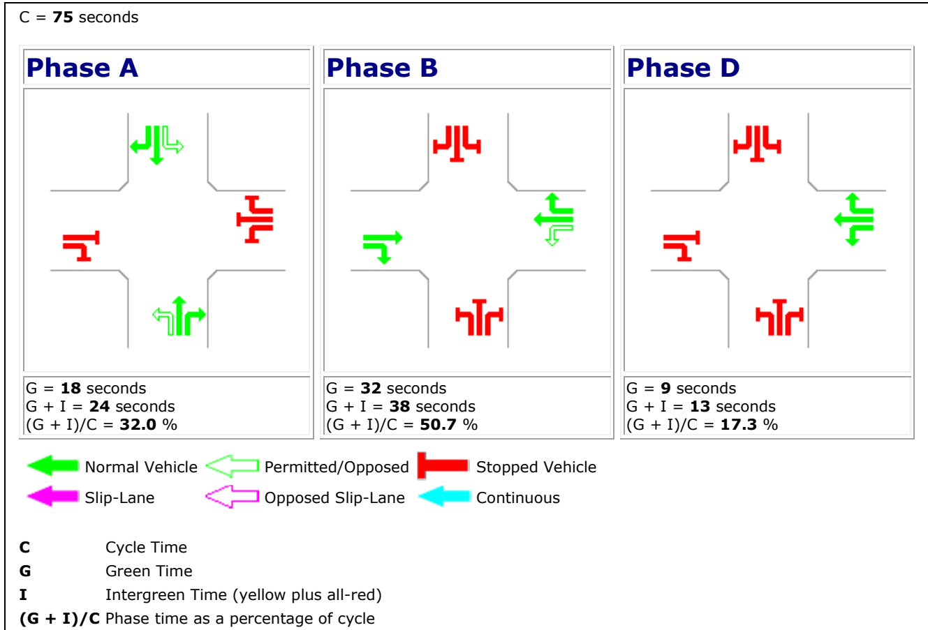
Figura 8-10: Nodo Viale dell'Industria-Viale del Commercio Fasatura impianto semaforico - Stato di Progetto
