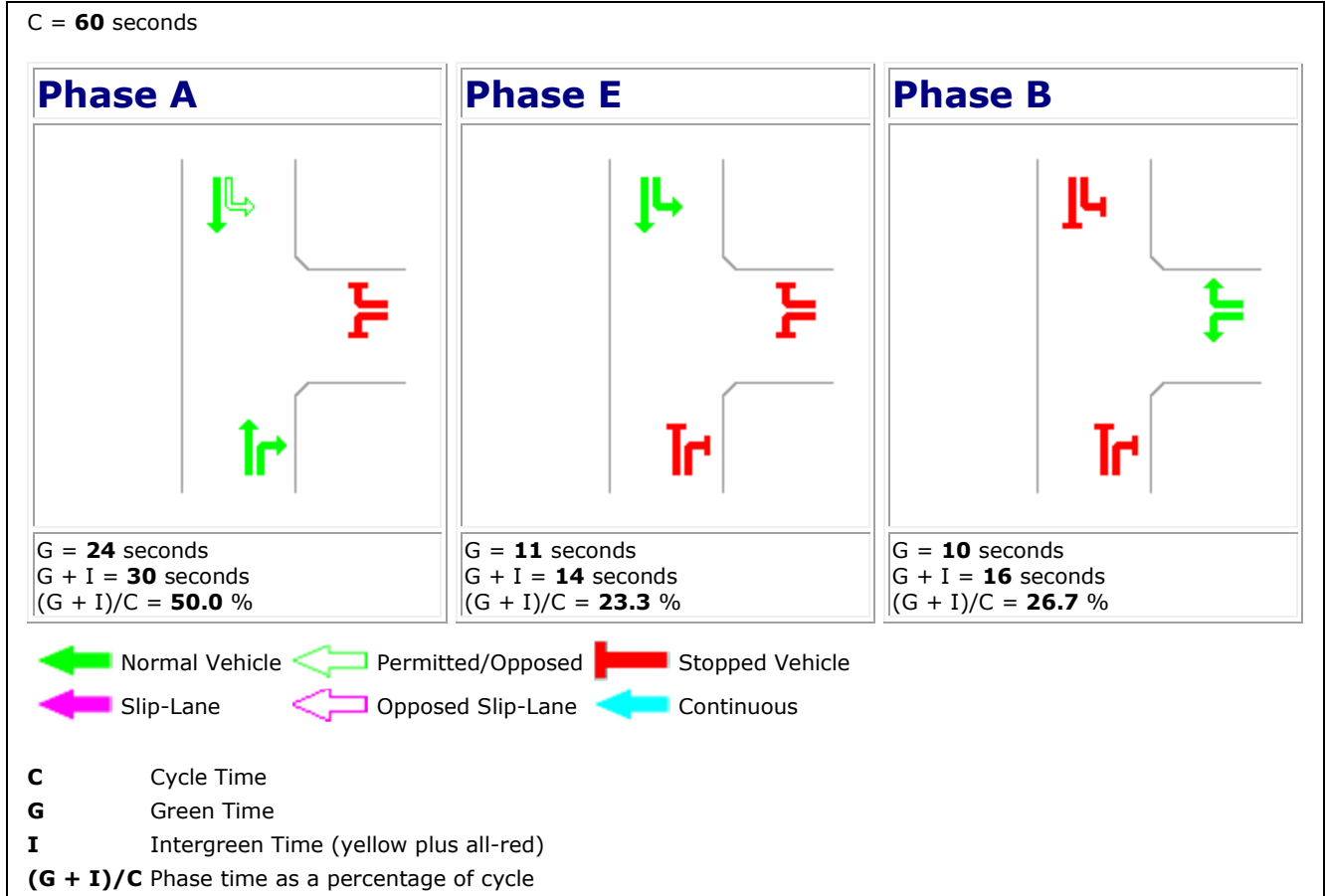
Figura 8-24: Nodo Nodo Via Santa Teresa-Via Molinara Fasatura impianto semaforico - Stato di Progetto
