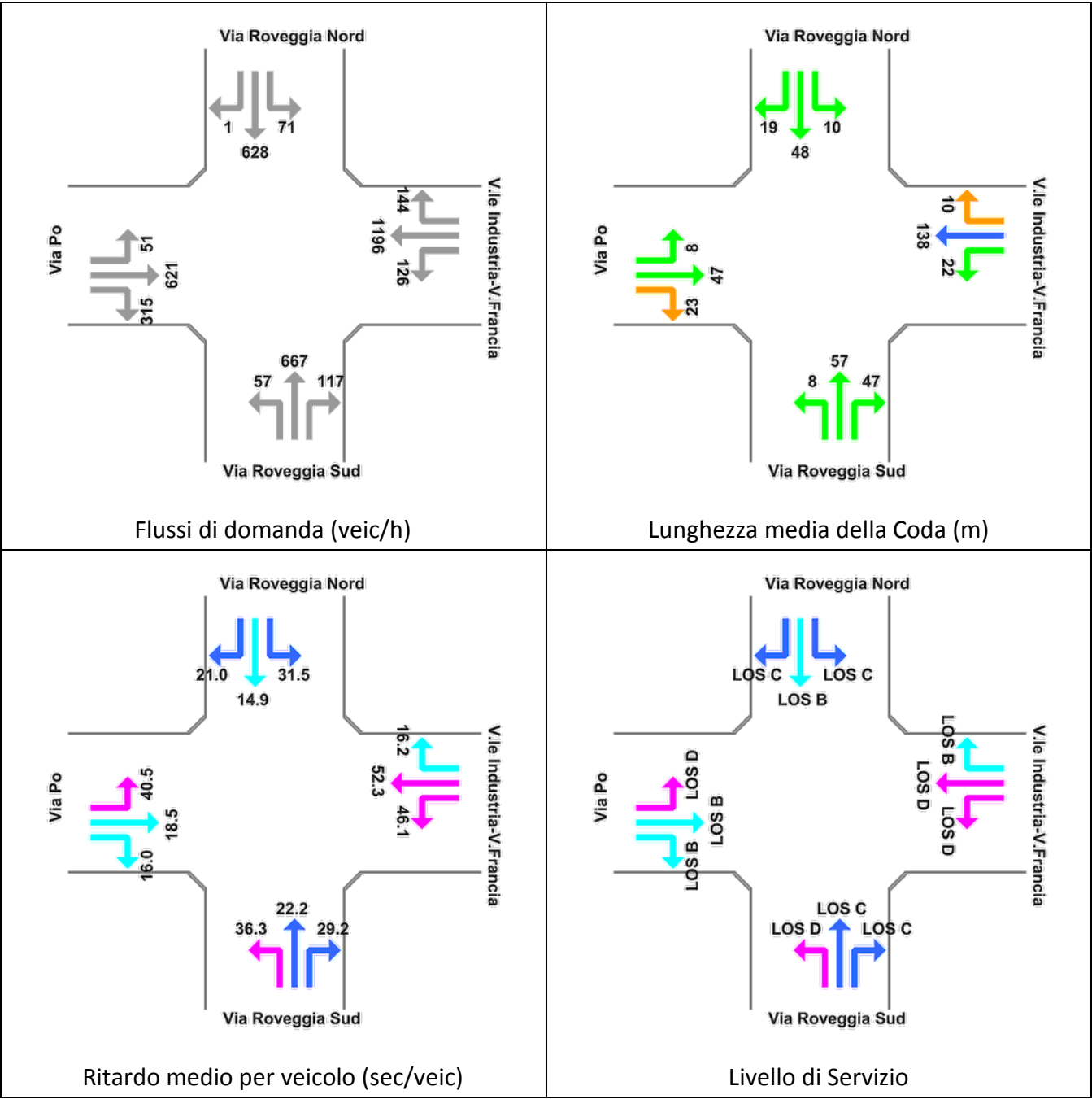
Figura 8-44: Nodo Via Roveggia-Viale dell'Industria-Via Po Risultati delle verifiche - Stato di Fatto Ora di Punta Venerdi 17.00-18.00
