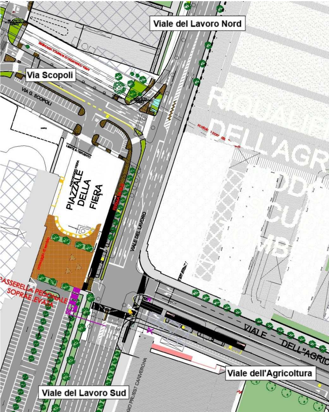
Figura 8-15: Nodo Viale del Lavoro-Viale dell'Agricoltura-Via Scopoli - Stato di Progetto
