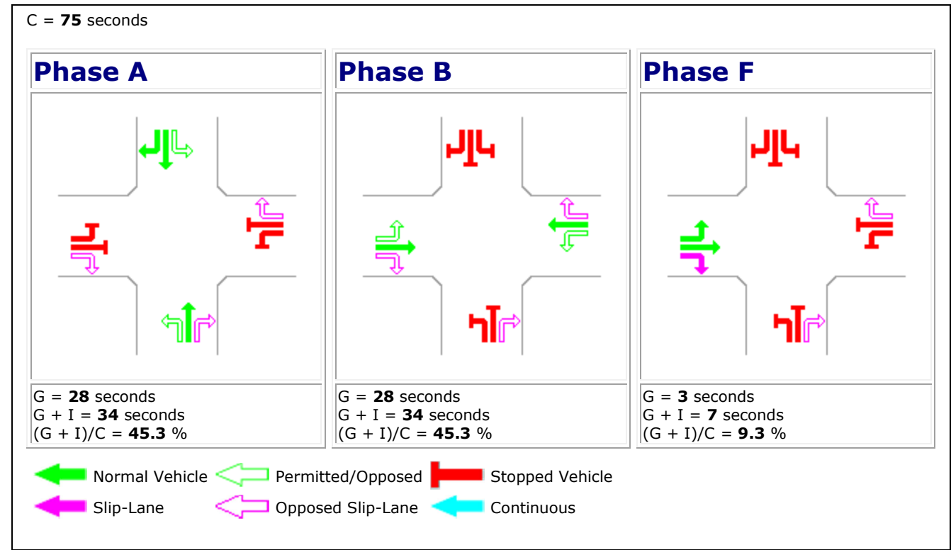
Figura 8-50: Nodo Via Roveggia-Via Scopoli-Via Murari Brà Fasatura impianto semaforico - Stato di Progetto
