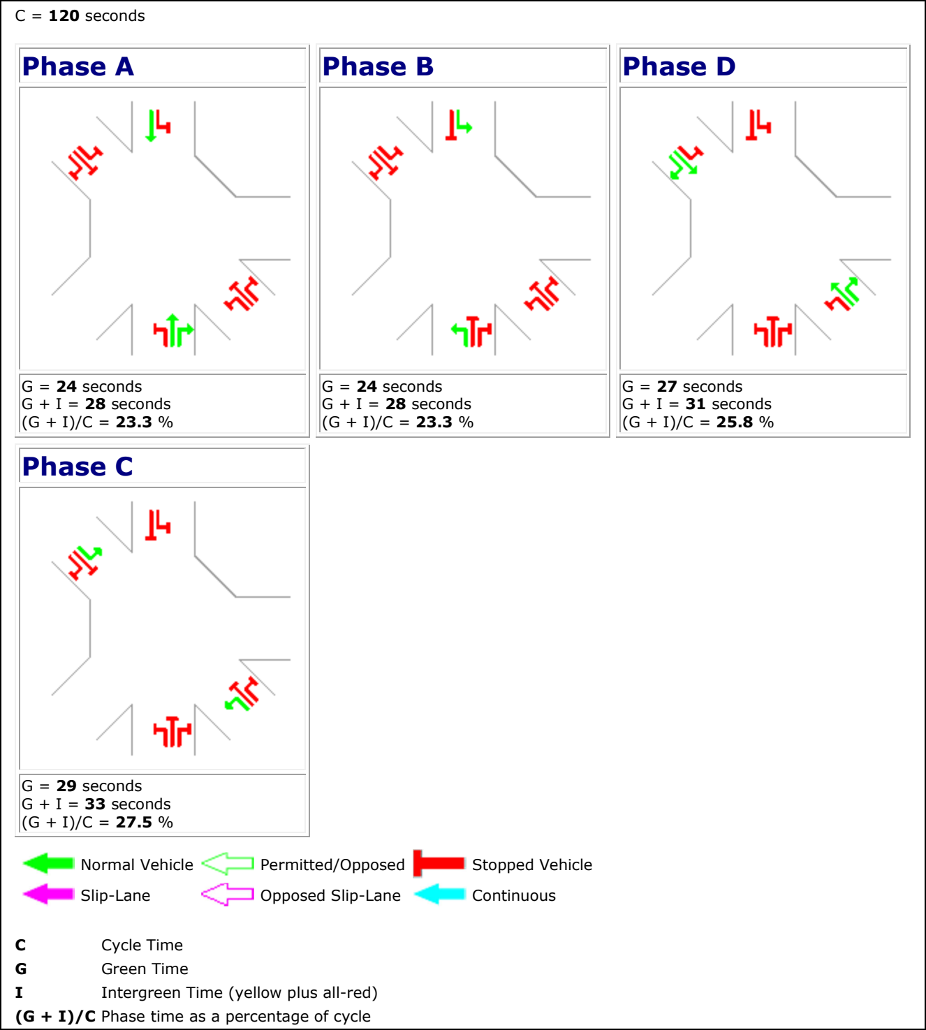
Figura 8-35: Nodo Via San Giacomo-Via Volturmo-Via Centro Fasatura impianto semaforico - Stato di Progetto
