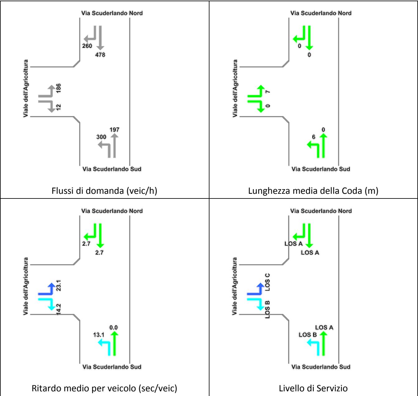
Figura 8-19: Nodo Viale dell'Agricoltura-Via Scuderlando Risultati delle verifiche - Stato di Fatto Ora di Punta Venerdì 17.00-18.00
