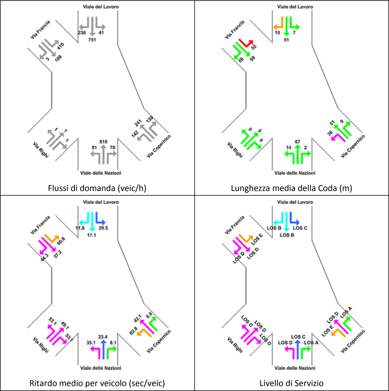
Figura 8-39: Nodo di Largo Perlar Risultati delle verifiche - Stato di Fatto Ora di Punta Venerdì 17.00-18.00
