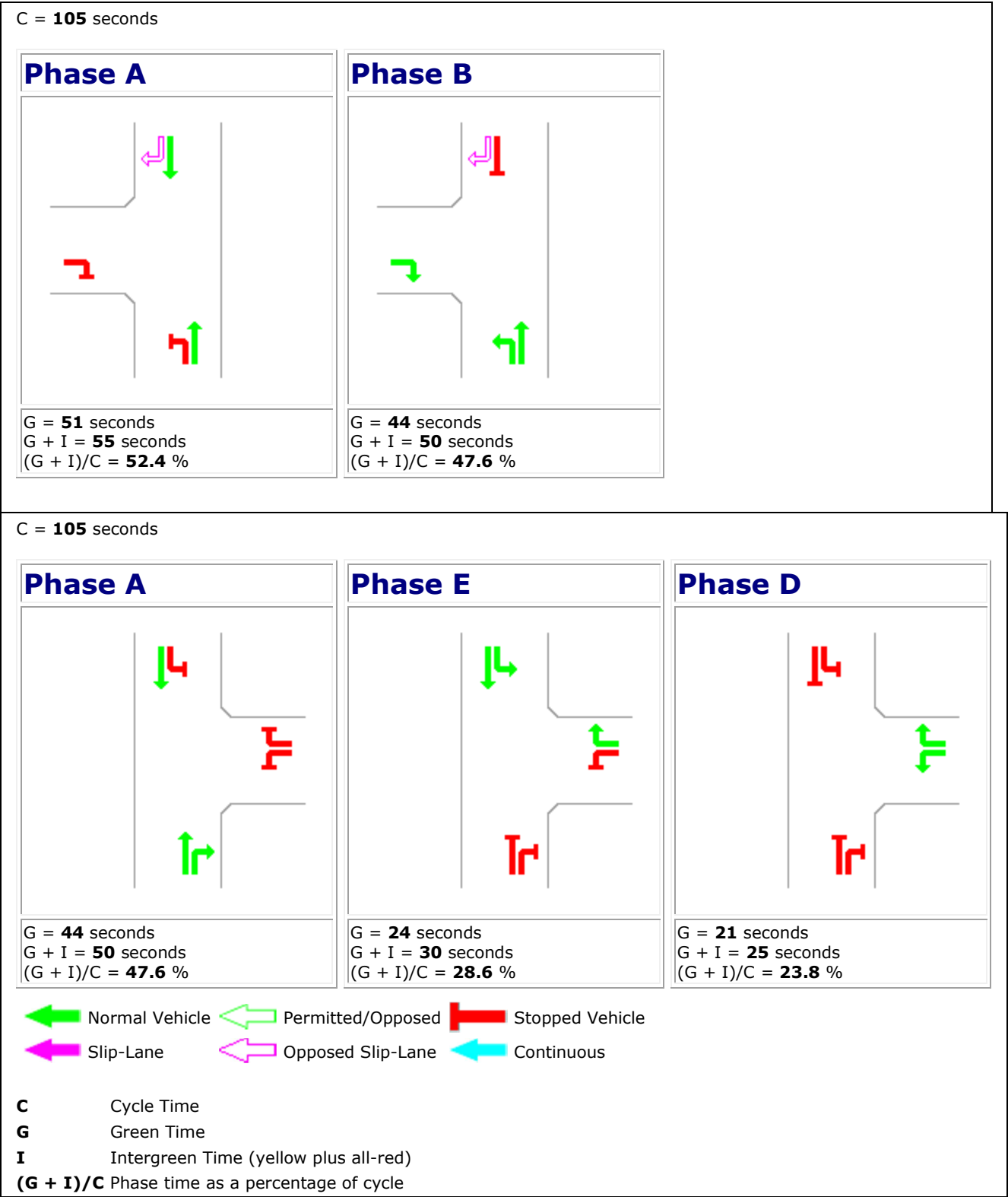
Figura 8-16: Nodo Viale del Lavoro-Viale dell'Agricoltura-Via Scopoli Fasatura impianto semaforico - Stato di Progetto
