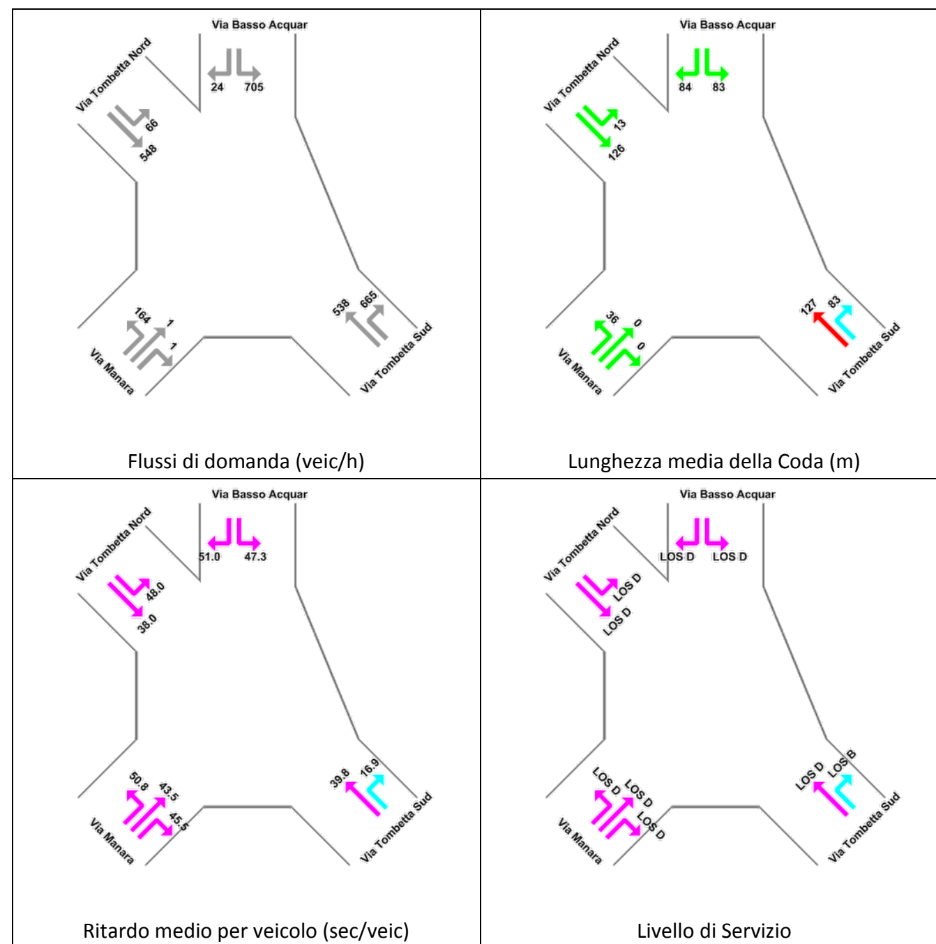
Figura 8-28: Nodo Via Tombetta-Via Basso Acquar Risultati delle verifiche - Stato di Fatto Ora di Punta Venerdì 17.00-18.00
