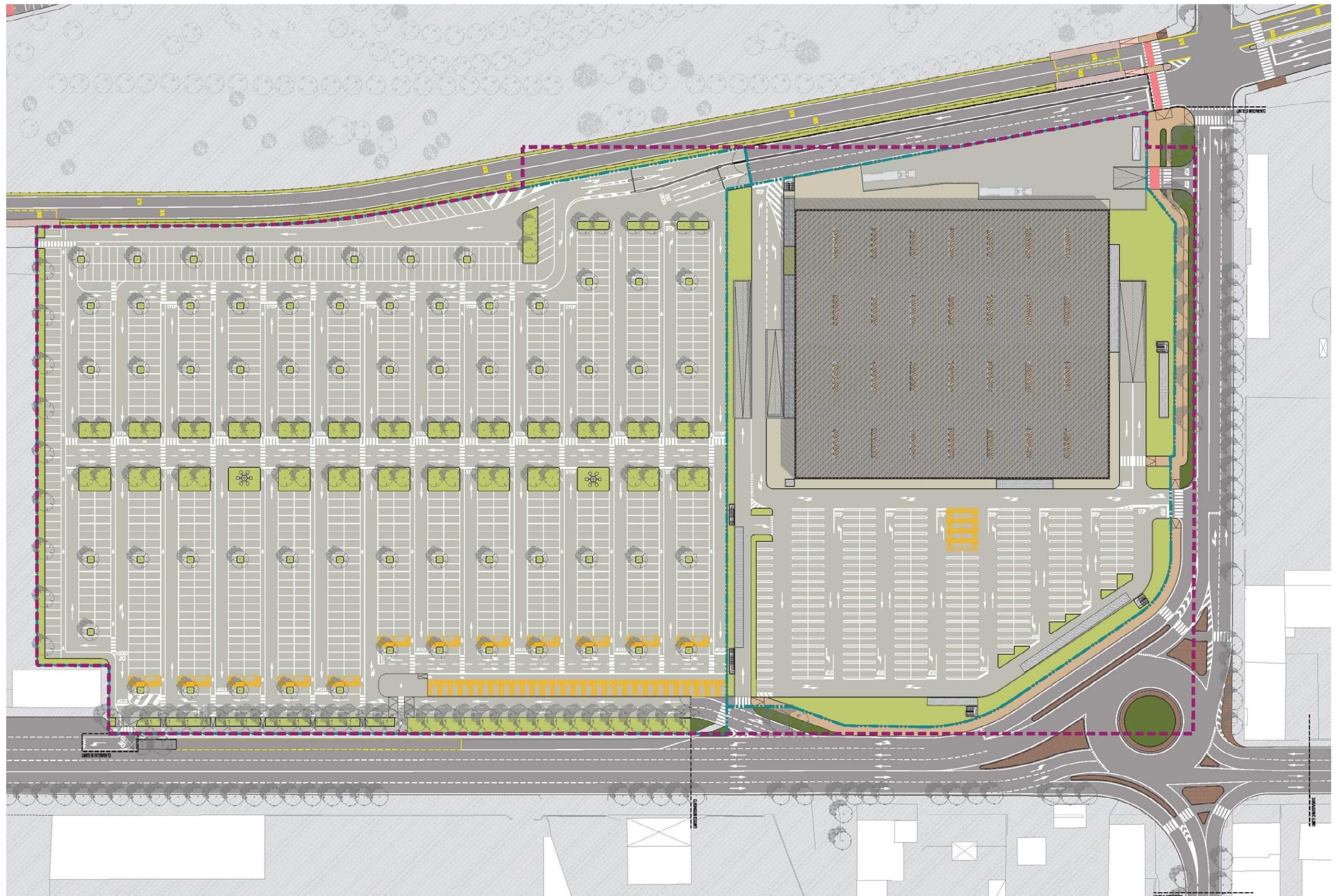
Figura 10-1: Planimetria Stato di Progetto - Polo Fieristico Veronese
