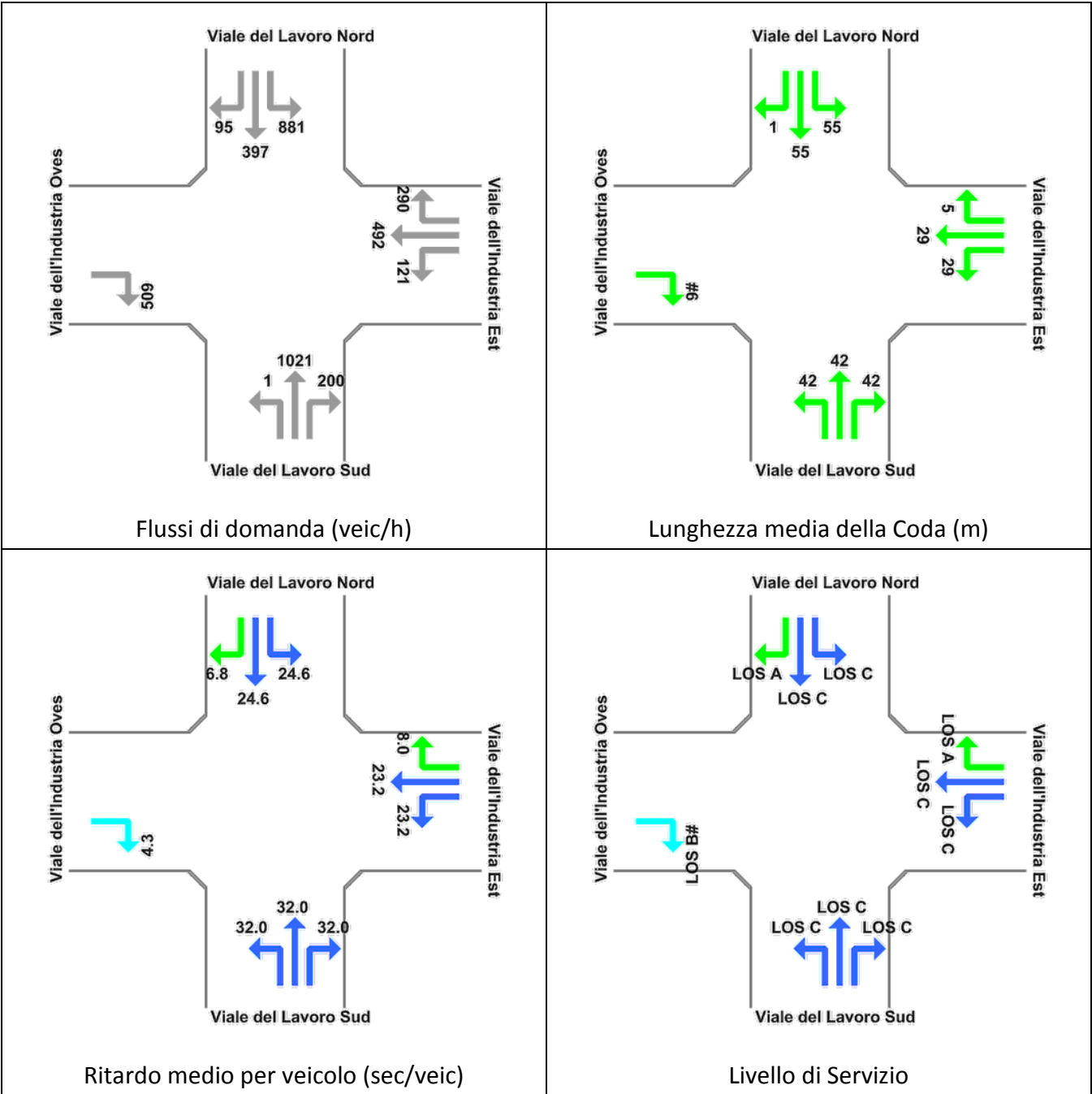
Figura 8-6: Nodo Viale del Lavoro-Viale dell'Industria Risultati delle verifiche - Stato di Progetto Ora di Punta Venerdì 17.00-18.00
