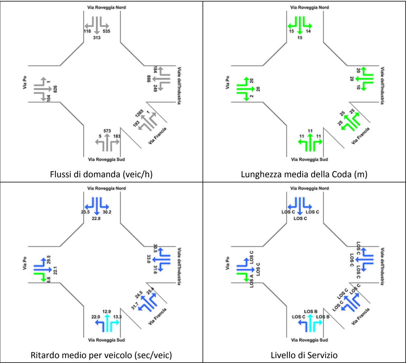
Figura 8-46: Nodo Via Roveggia-Viale dell'Industria-Via Po Risultati delle verifiche - Stato di Progetto Ora di Punta Venerdi 17.00-18.00
