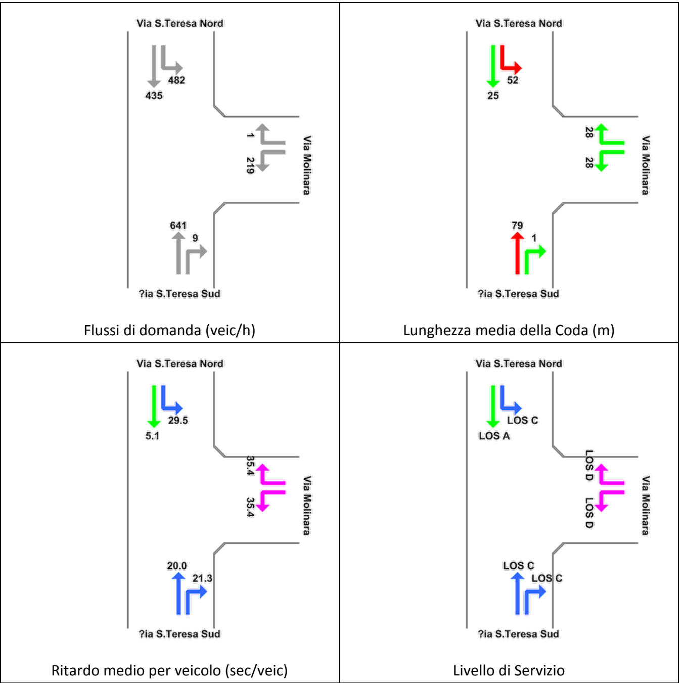
Figura 8-25: Nodo Via Santa Teresa-Via Molinara Risultati delle verifiche - Stato di Progetto Ora di Punta Venerdì 17.00-18.00
