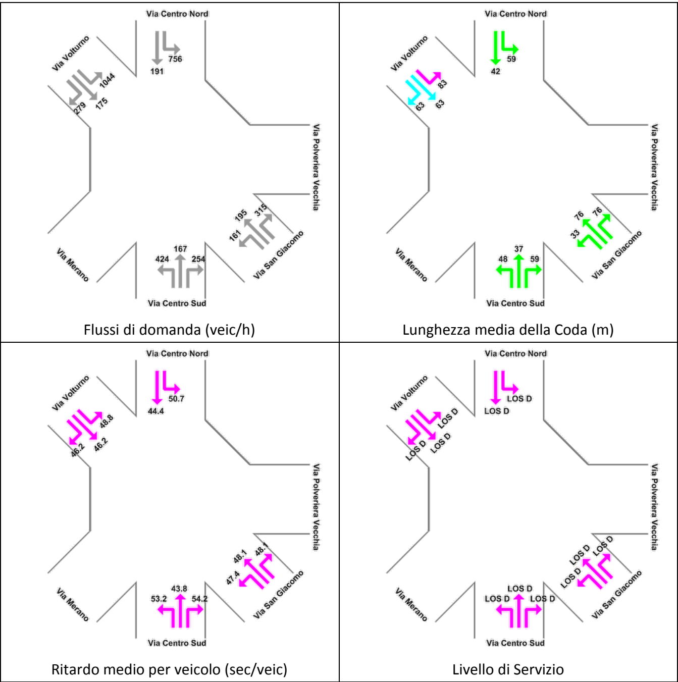
Figura 8-36: Nodo Via San Giacomo-Via Volturmo-Via Centro Risultati delle verifiche - Stato di Progetto Ora di Punta Venerdì 17.00-18.00
