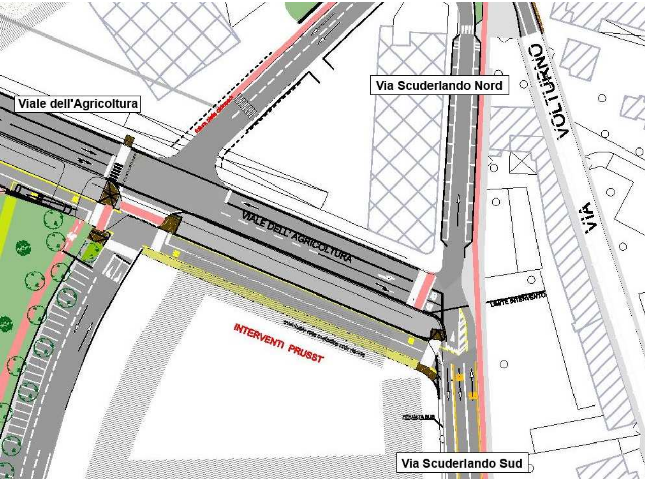
Figura 8-20: Nodo Viale dell'Agricoltura-Via Scuderlando - Stato di Progetto
