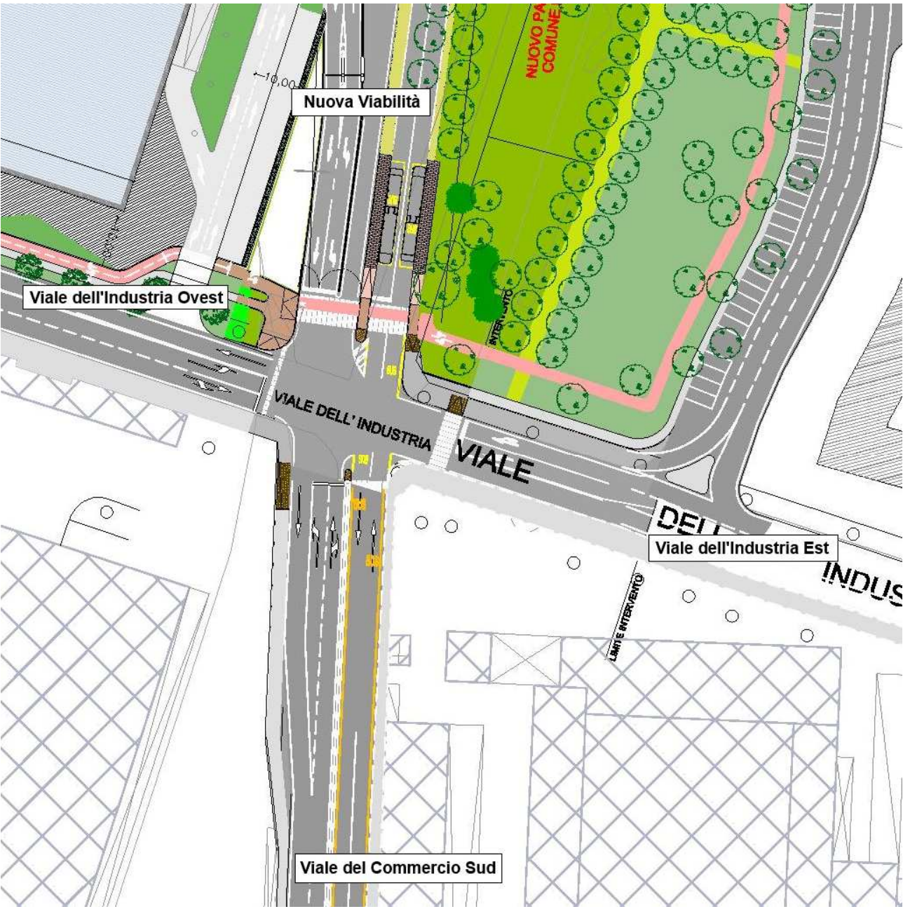
Figura 8-9: Nodo Viale dell'Industria-Viale del Commercio - Stato di Progetto
