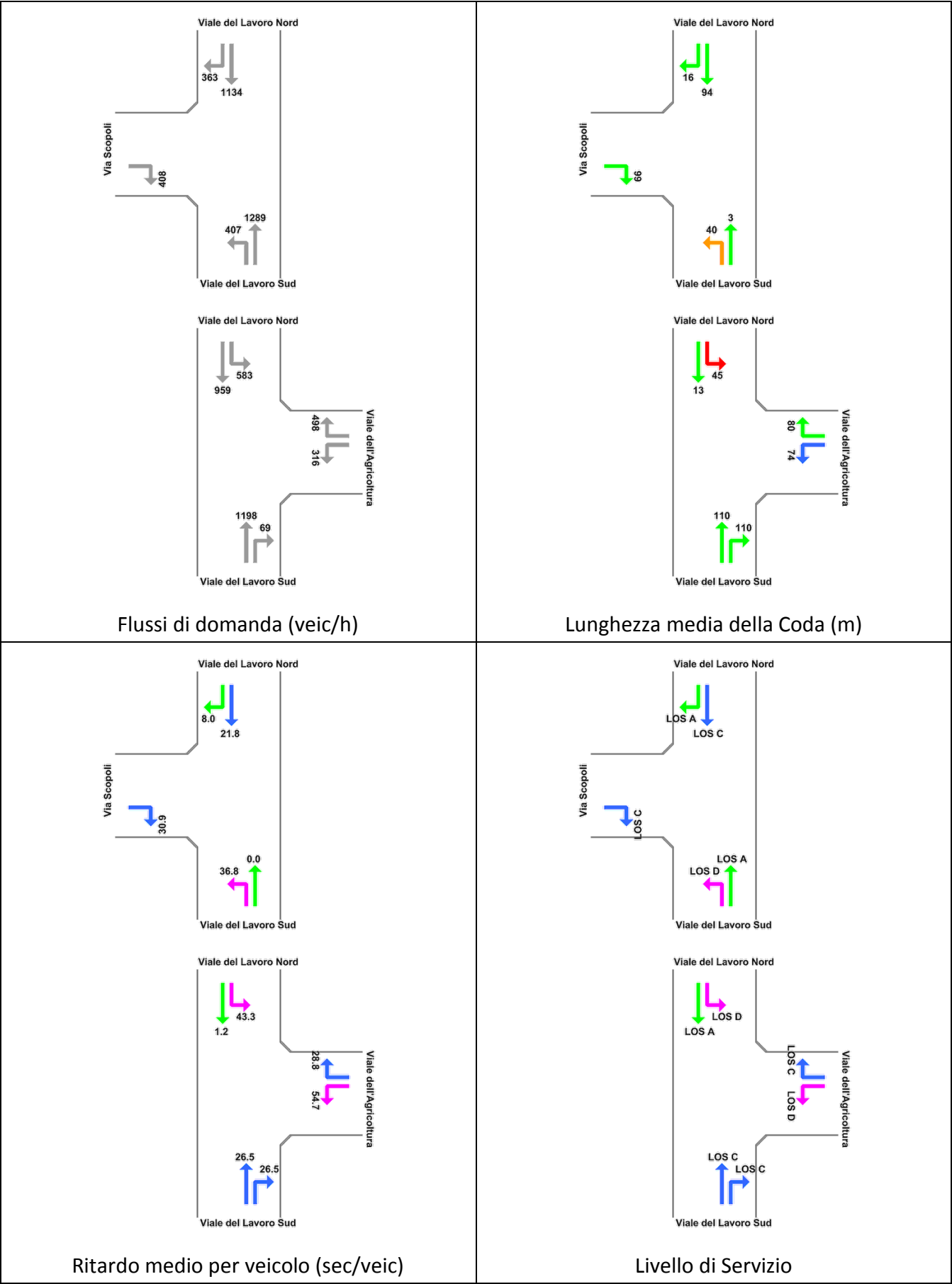
Figura 8-17: Nodo Viale del Lavoro-Viale dell'Agricoltura-Via Scopoli Risultati delle verifiche - Stato di Progetto Ora di Punta Venerdì 17.00-18.00
