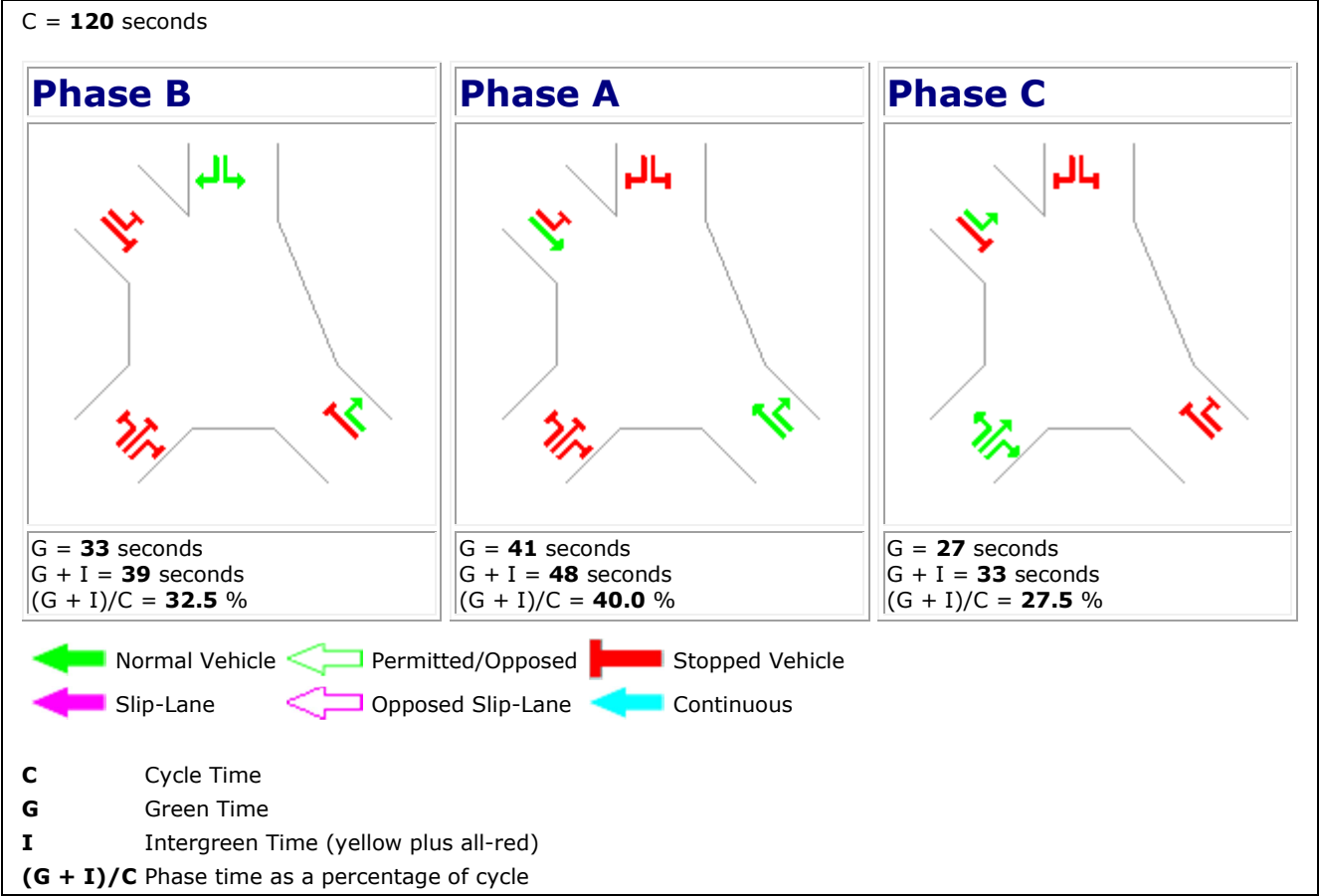
Figura 8-27: Nodo Via Tombetta-Via Basso Acquar Fasatura impianto semaforico - Stato di Fatto
