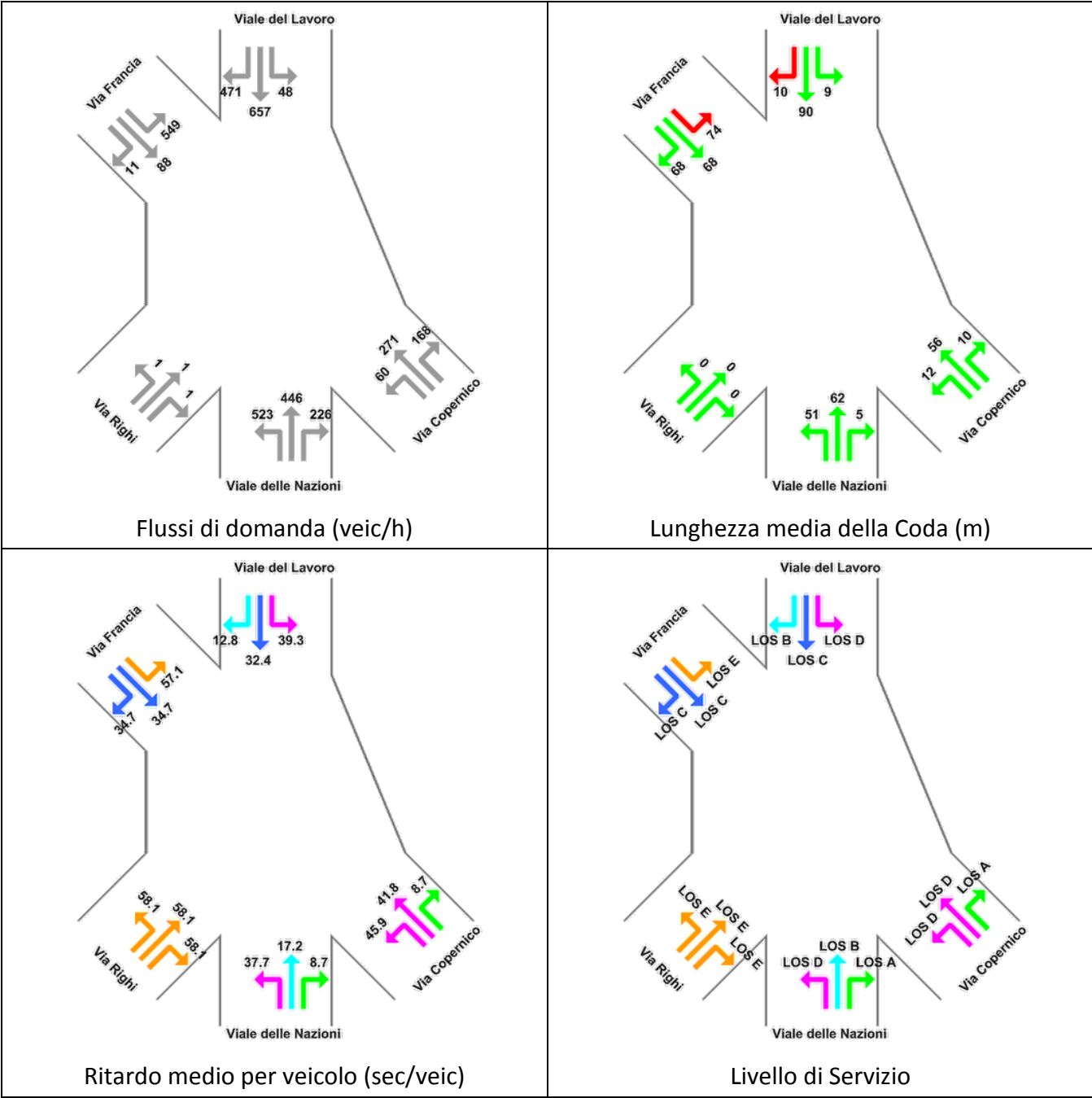
Figura 8-41: Nodo di Largo Perlar Risultati delle verifiche - Stato di Progetto Ora di Punta Venerdì 17.00-18.00
