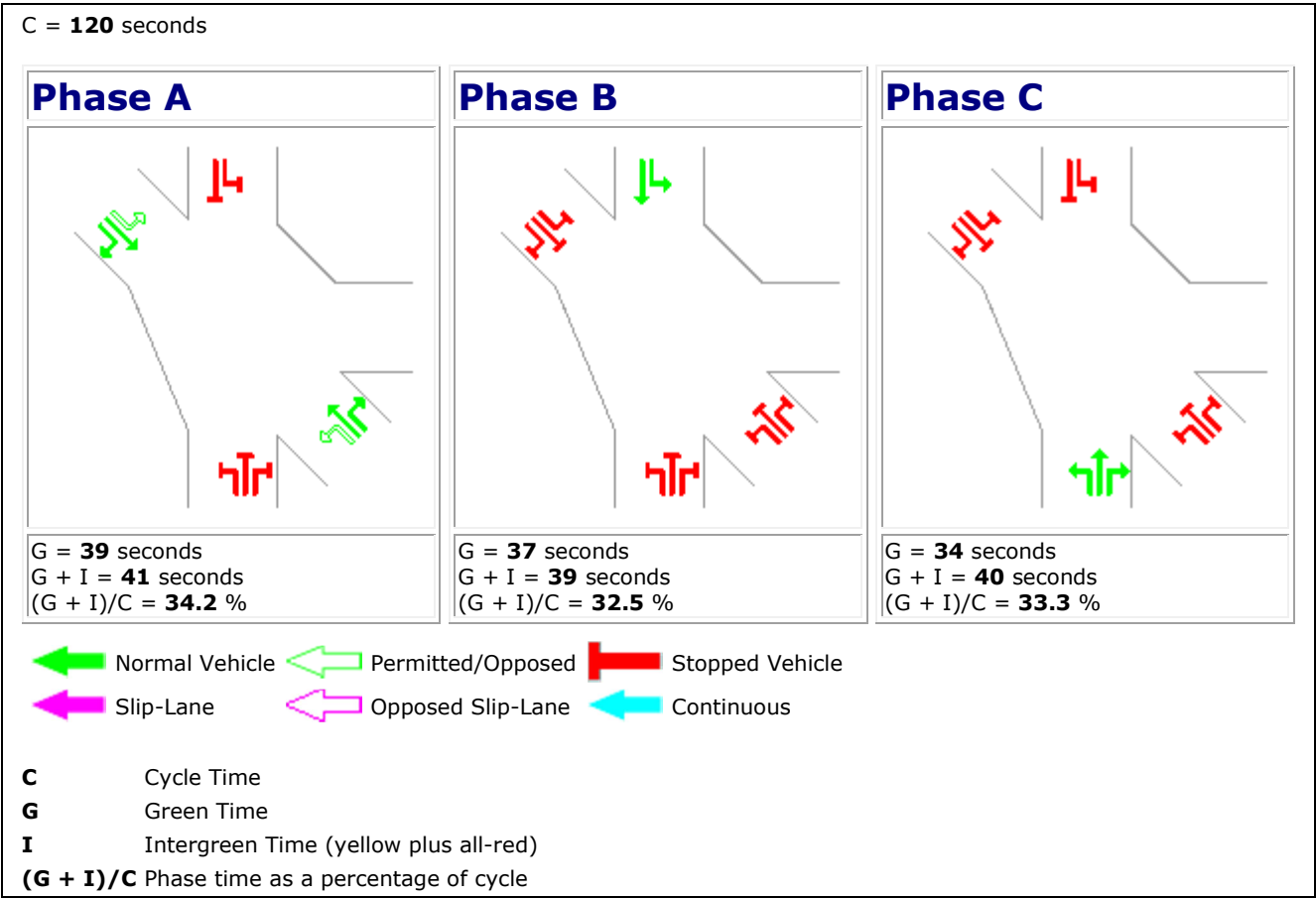
Figura 8-33: Nodo Via San Giacomo-Via Volturno-Via Centro Fasatura impianto semaforico - Stato di Fatto
