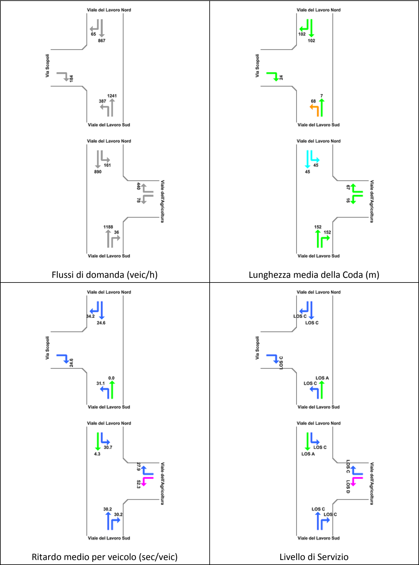
Figura 8-14: Nodo Viale del Lavoro-Viale dell'Agricoltura-Via Scopoli Risultati delle verifiche - Stato di Fatto Ora di Punta Venerdì 17.00-18.00
