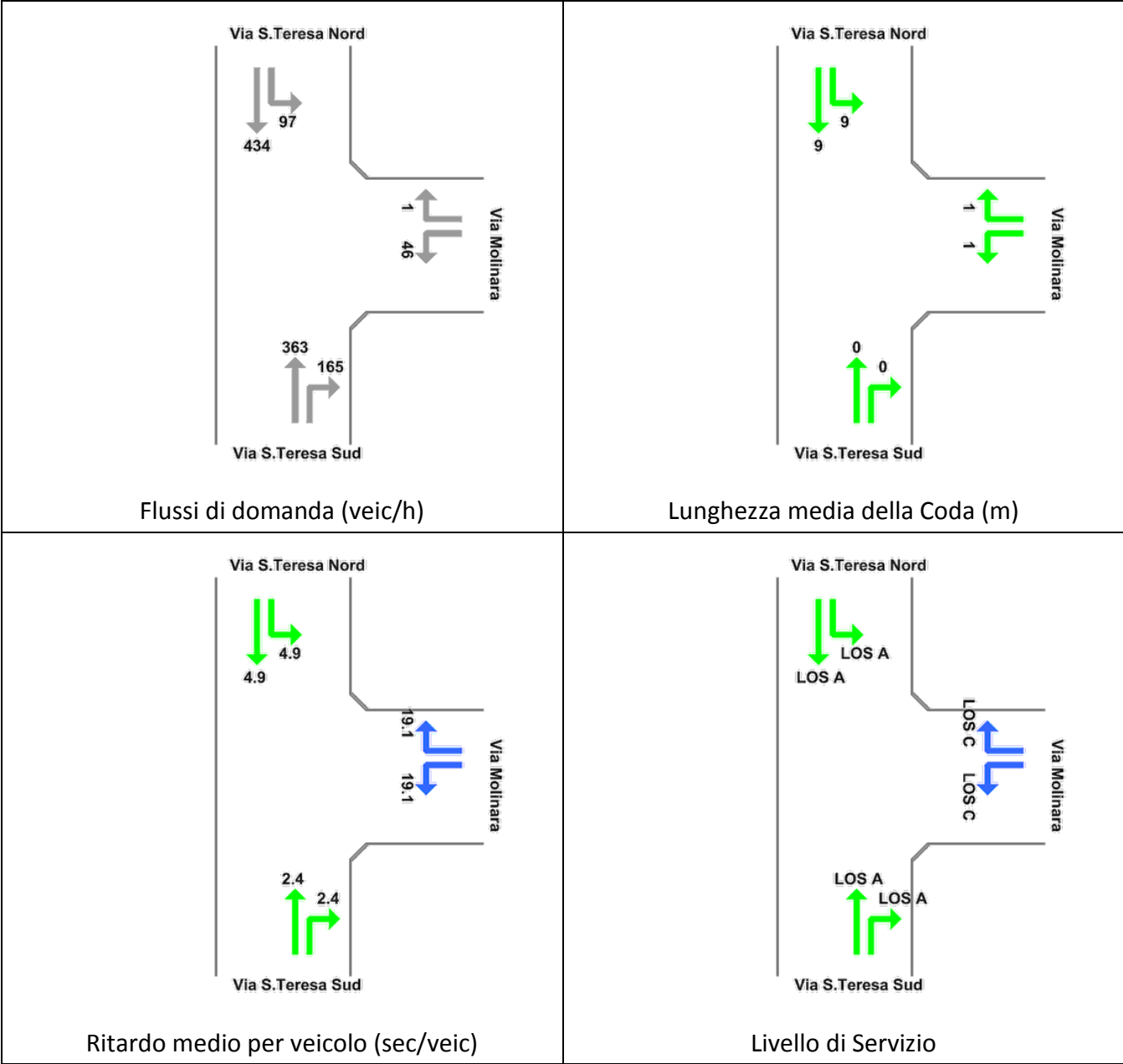
Figura 8-22: Nodo Via Santa Teresa-Via Molinara Risultati delle verifiche - Stato di Fatto Ora di Punta Venerdì 17.00-18.00
