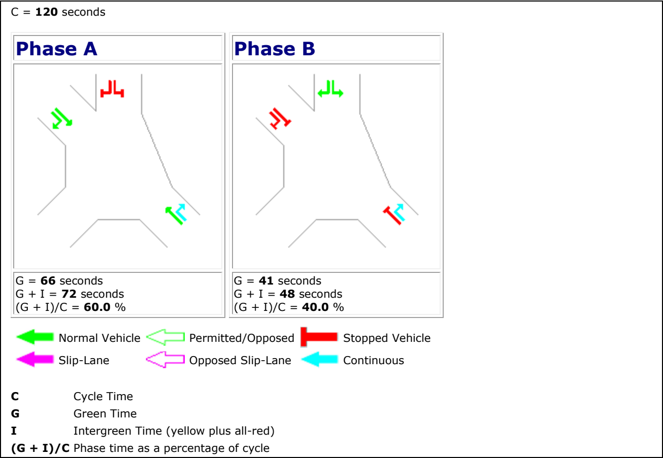
Figura 8-30: Nodo Via Tombetta-Via Basso Acquar Fasatura impianto semaforico - Stato di Progetto
