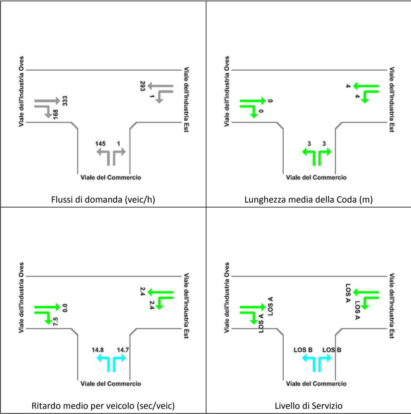
Figura 8-8: Nodo Viale dell'Industria-Viale del Commercio Risultati delle verifiche - Stato di Fatto Ora di Punta Venerdì 17.00-18.00
