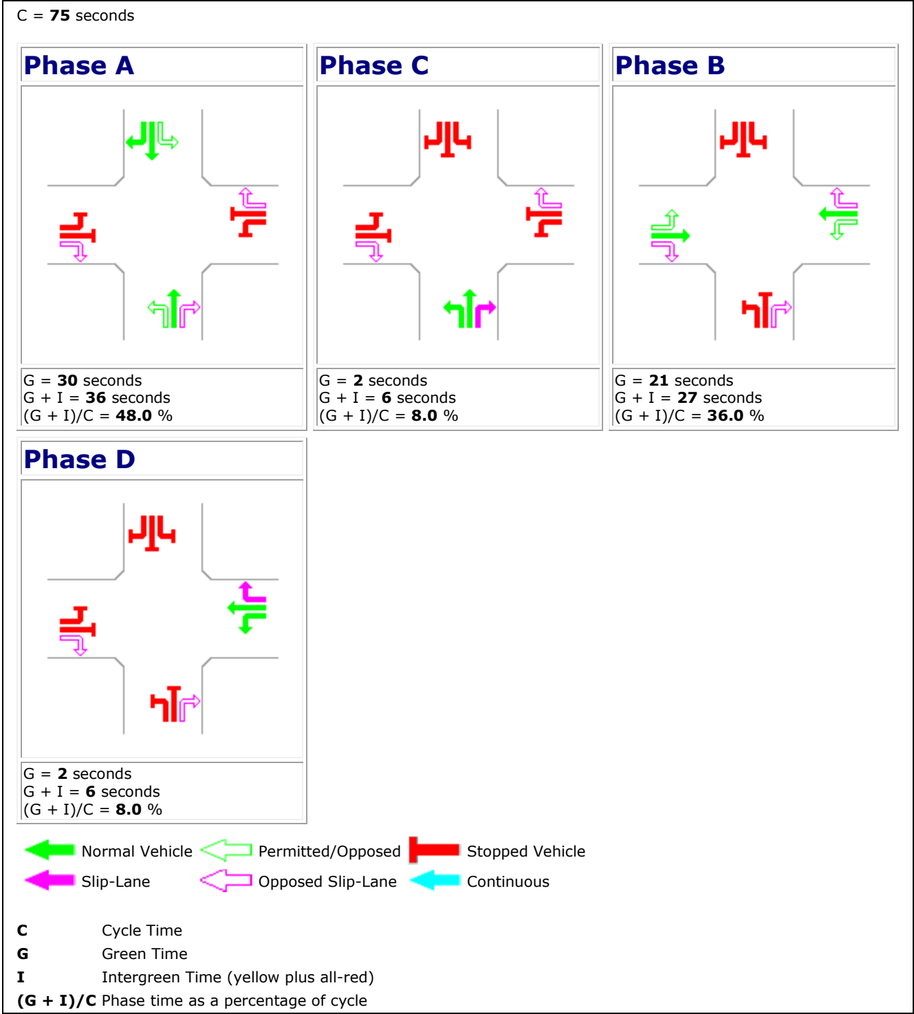
Figura 8-48: Nodo Via Roveggia-Via Scopoli-Via Murari Brà Fasatura impianto semaforico - Stato di Fatto
