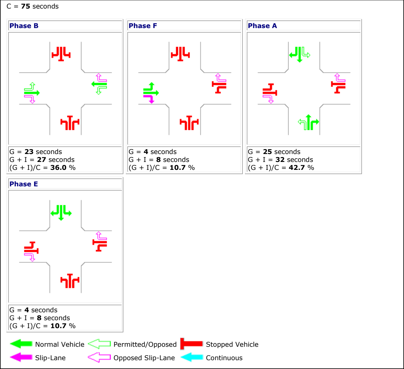
Figura 8-43: Nodo Via Roveggia-Viale dell'Industria-Via Po Fasatura impianto semaforico - Stato di Fatto
