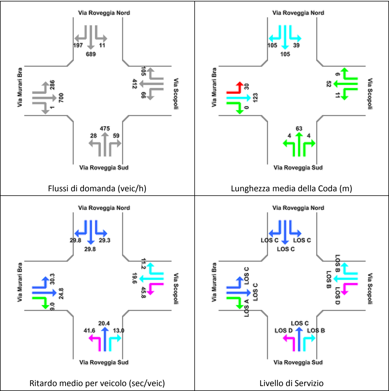
Figura 8-51: Nodo Via Roveggia-Via Scopoli-Via Murari Brà Risultati delle verifiche - Stato di Progetto Ora di Punta Venerdì 17.00-18.00
