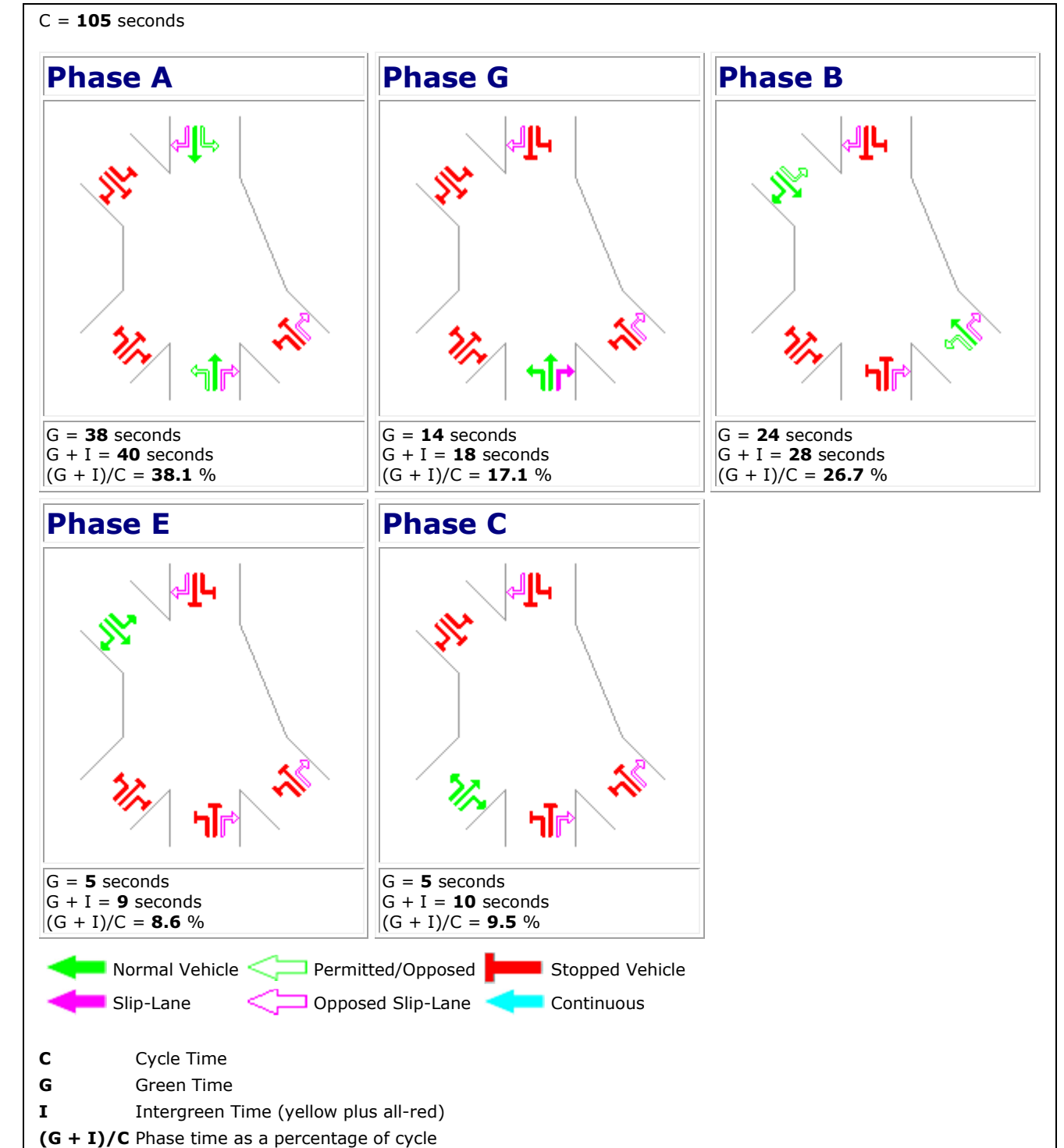
Figura 8-40: Nodo di Largo Perlar Fasatura impianto semaforico - Stato di Progetto
