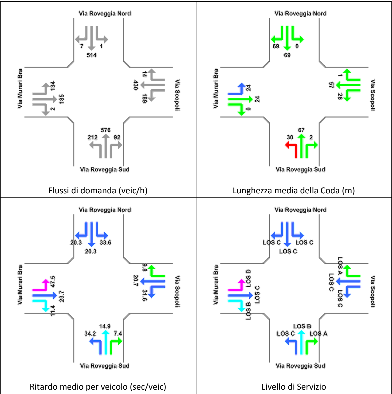
Figura 8-49: Nodo Via Roveggia-Via Scopoli-Via Murari Brà Risultati delle verifiche - Stato di Fatto Ora di Punta Venerdì 17.00-18.00
