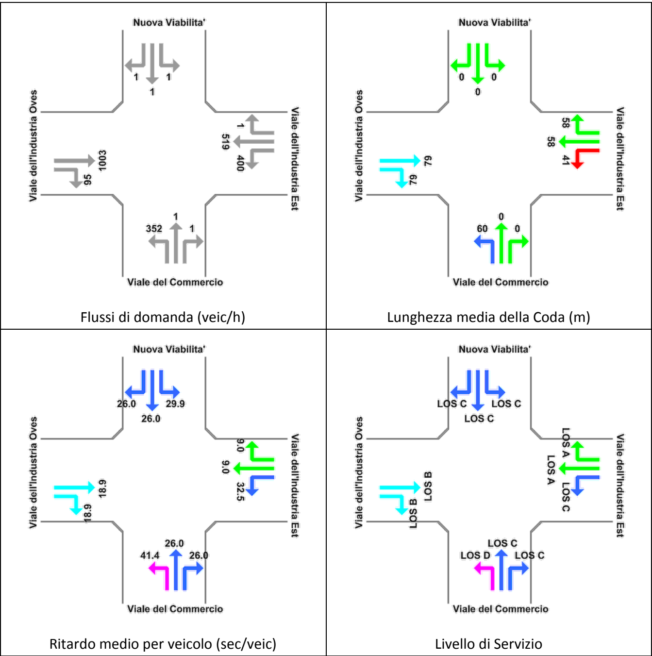
Figura 8-11: Nodo Viale dell'Industria-Viale del Commercio Risultati delle verifiche - Stato di Progetto Ora di Punta Venerdì 17.00-18.00
