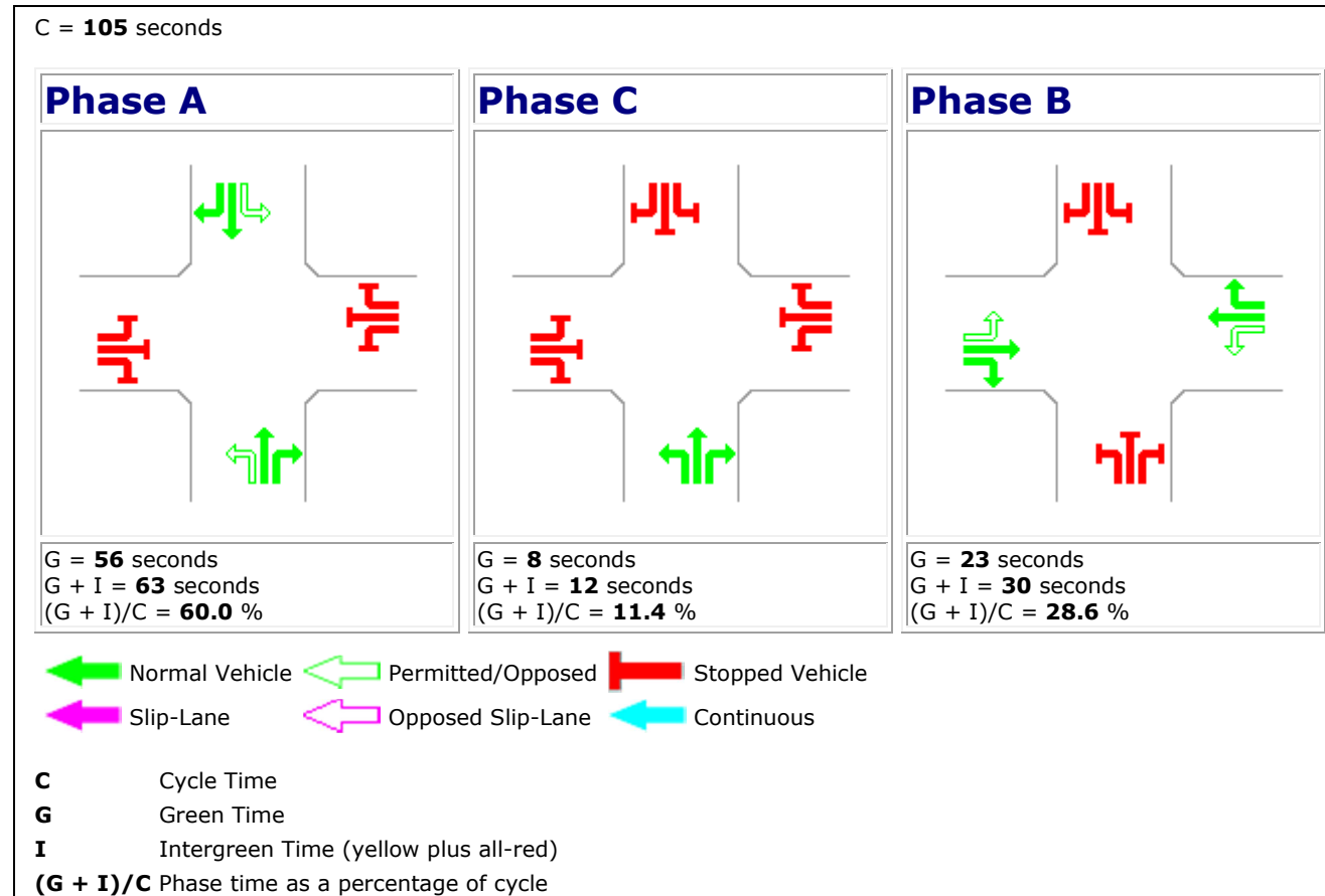
Figura 8-3: Nodo Viale del Lavoro-Viale dell'Industria Fasatura impianto semaforico - Stato di Fatto
